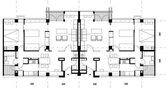
Originalni projekat dve tipske stambene jedinice br. 1
