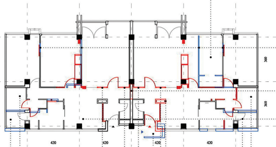
Preklapljeni planovi uklonjenih i dodatih pregrada i otvora
