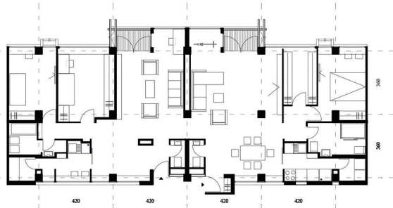
Trenutno stanje dve tipske stambene jedinice br. 1 (spojene u jednu novu stambenu jedinicu)
