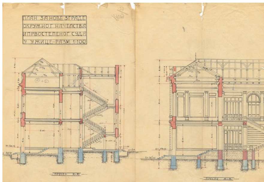
Слика 14. Пресек А-Б и пресек К-М
