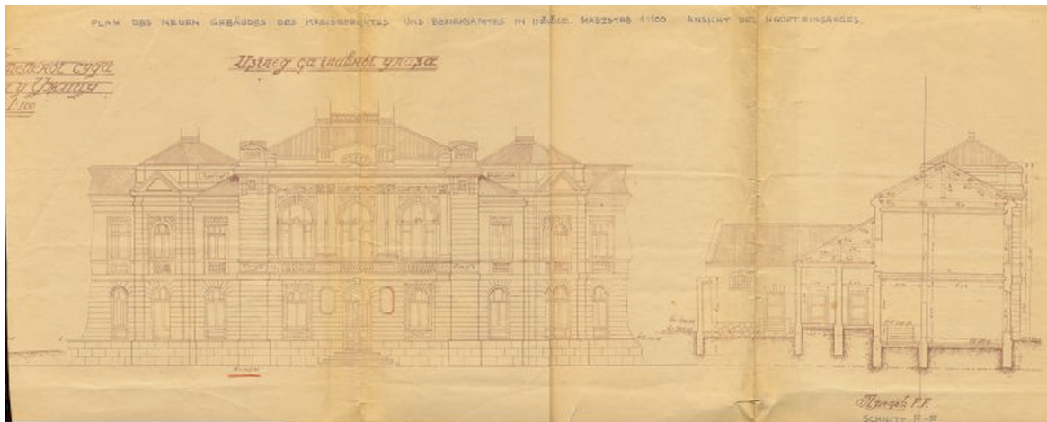
Слика 16. Изглед са главног улаза Figure 16. Layout from main entrance
