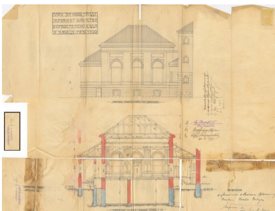
Слика 12. Изглед и пресек судске сале из дворишта
