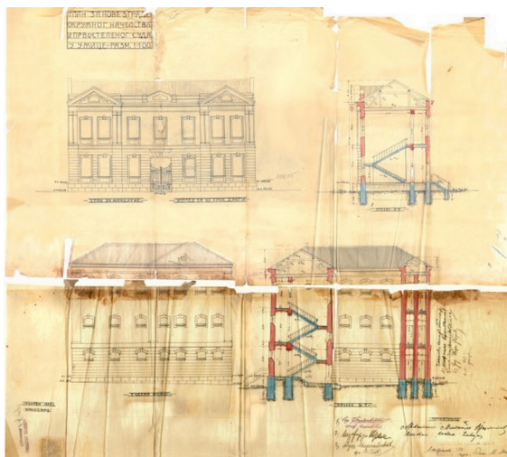
Слика 13. Стан за жандарме - изглед, пресек О-П, судска апсана и пресек С-Т
