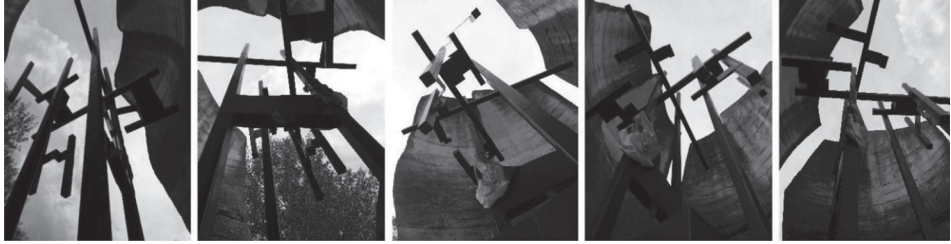
Сл. 12 Челична конструкција Споменика на Брезовици (фото Драган Николчевић)
