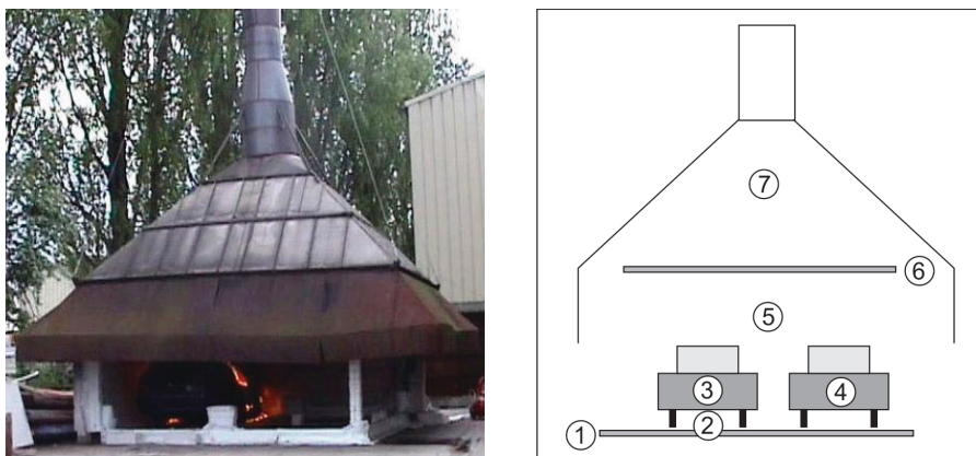
Slika 1: Realni izgled i šematski prikaz uslova eksperimenta: 1 – platforma za merenje gubitka mase, 2 – izvor paljenja, 3 – manje vozilo, 4 – veće vozilo, 5 – termoparovi za merenje temperature, 6 – tavanica na visini od 2,6 m, 7 – odvod produkata sagorevanja.
