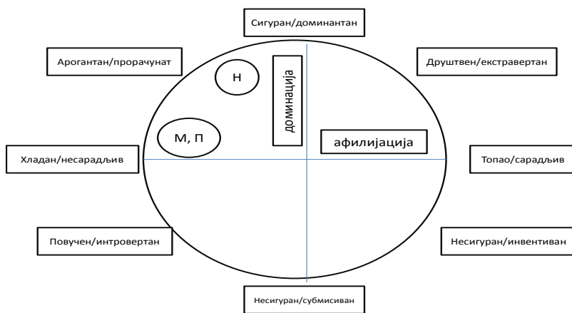
Слика 1. Интерперсонални циркумплексни модел и положај компоненти Мрачне тријаде унутар модела (в. KB2) (Wiggins, 1985)
