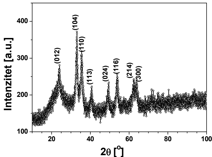
Slika 1 – Difraktogram nanočestičnog uzorka \alpha - Fe_2O_3/SiO_2 , dobijen rasejanjem X-zraka Figure 1 – X-ray powder diffraction pattern of the nanocomposite \alpha - Fe_2O_3/SiO_2
