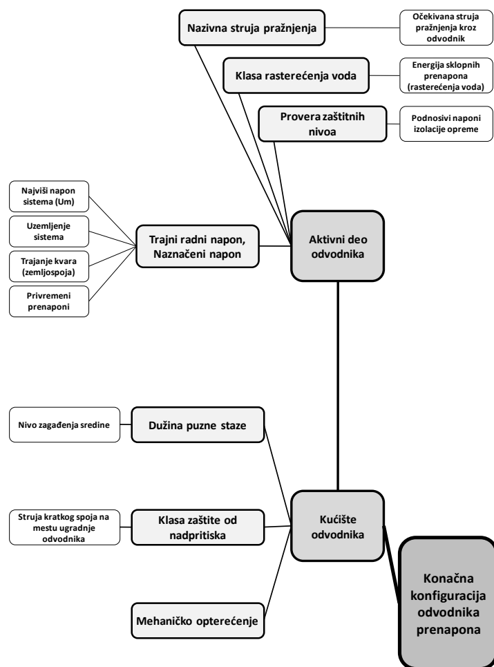
Slika 1. Blok dijagram generalnog postupka izbora odvodnika
