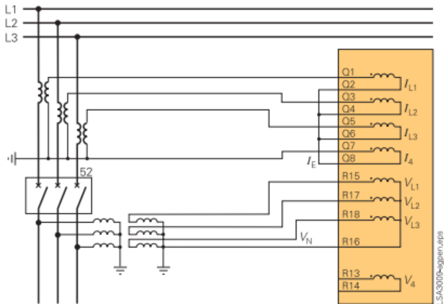
Слика 7: Шема везивања струјних трансформатора за усмерену земљоспојну и дистантну заштиту далековода
